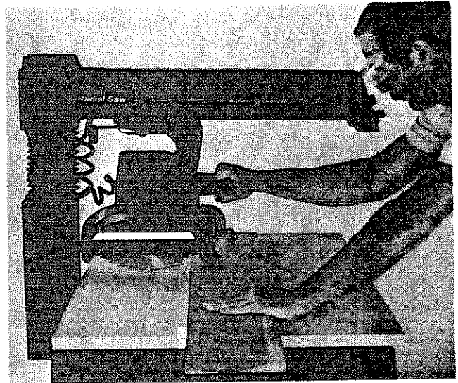
Fig. 83 Bevel Crosscut
