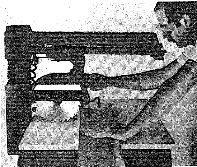
Fig. 81 Straight Crosscut
