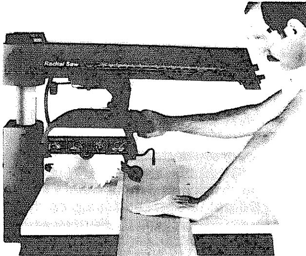
Fig. 81 - Straight Crosscut
