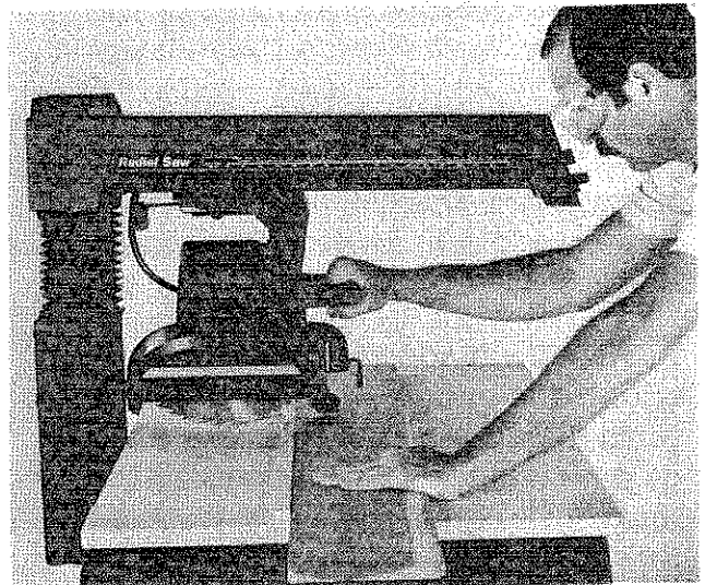
Fig. 83 - Bevel Crosscut
